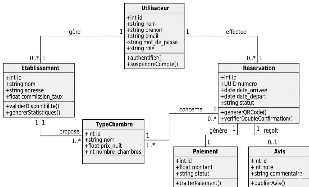
Figure 13: Diagramme d'entité relation en diagramme de classe
