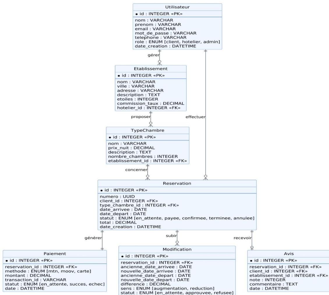
Figure 12: Diagramme d'entité relation
