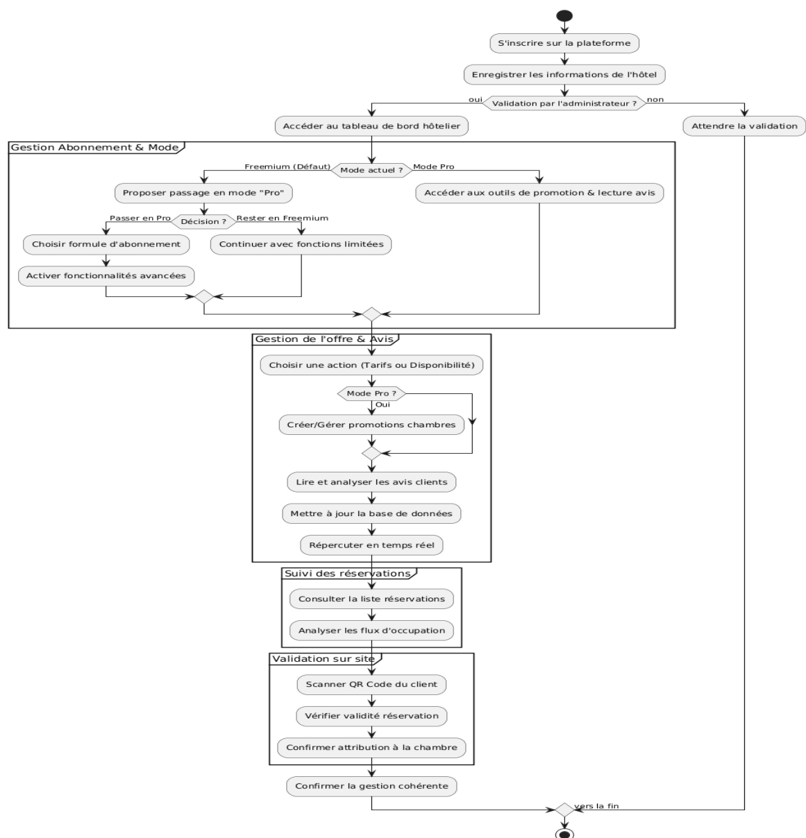
Figure 7: Diagramme d'état de cas gérer un établissement /hôtel
