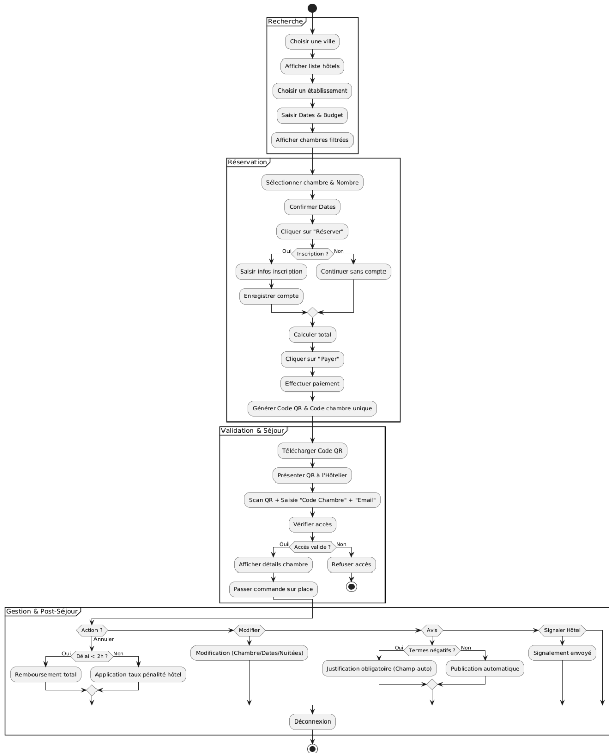
Figure 6: Diagramme d'état de cas gérer réservation
