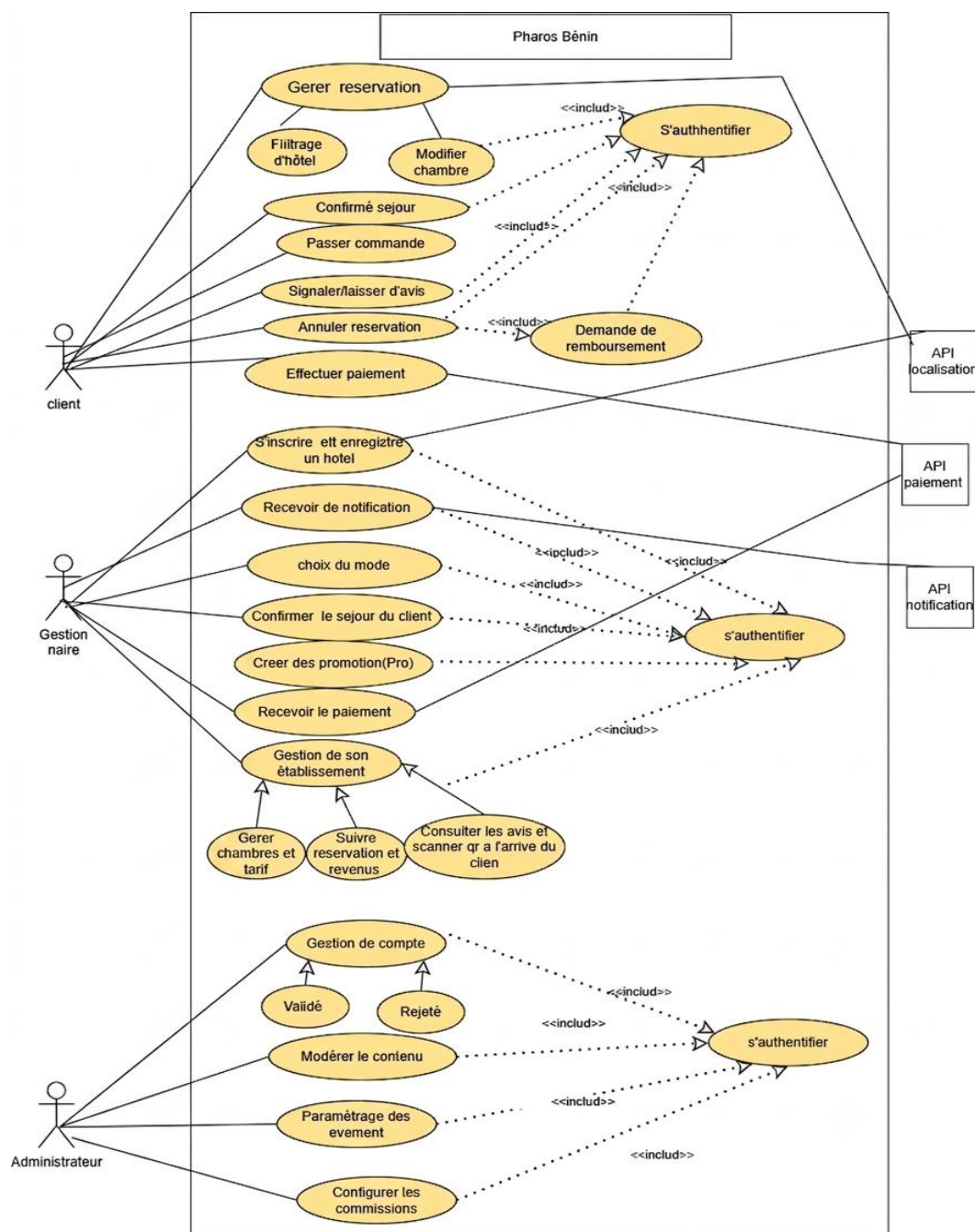
Figure 2: Diagramme de cas d'utilisation
