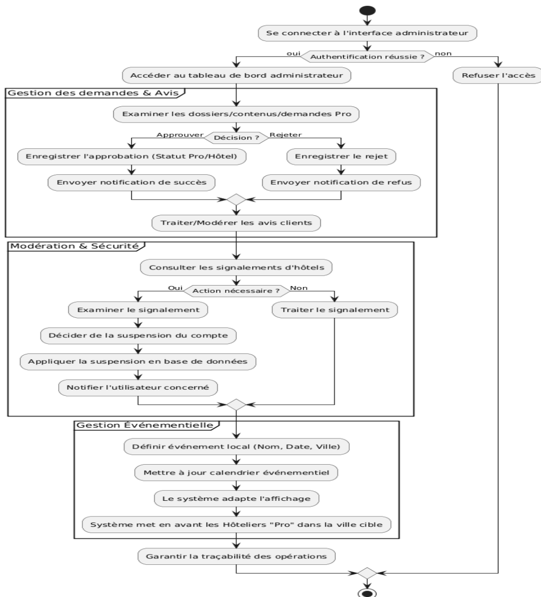
Figure 8 : Diagramme d'état de cas supervision et contrôle de la plateforme
