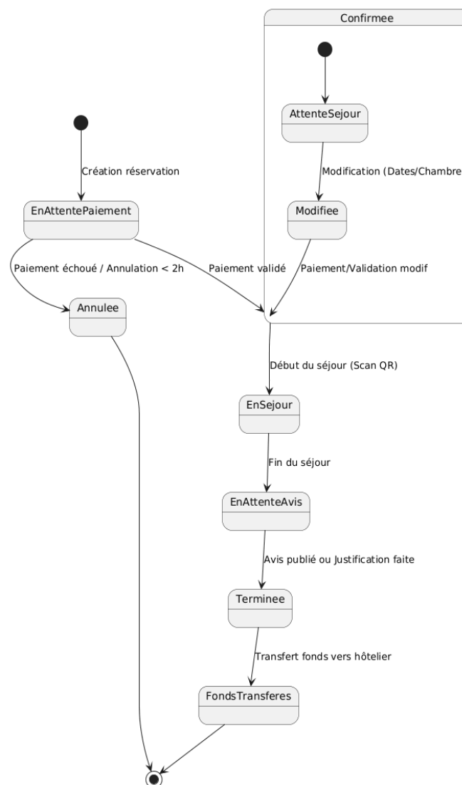
Figure 9: Diagramme d'état de cas gérer réservation
