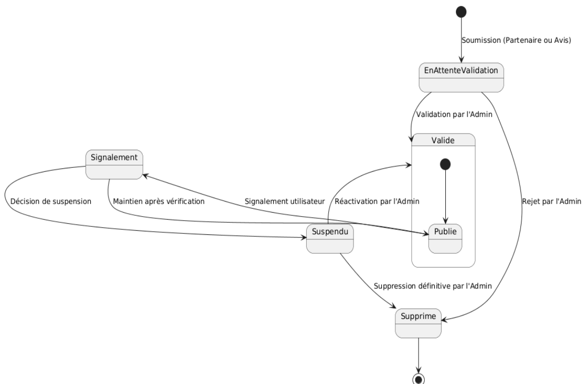
Figure 11: Diagramme d'état de cas Supervision et contrôle de la plateforme.
