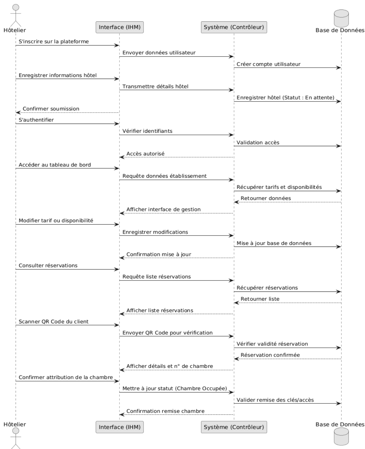
Figure 4: Diagramme de séquences de cas gérer un établissement
