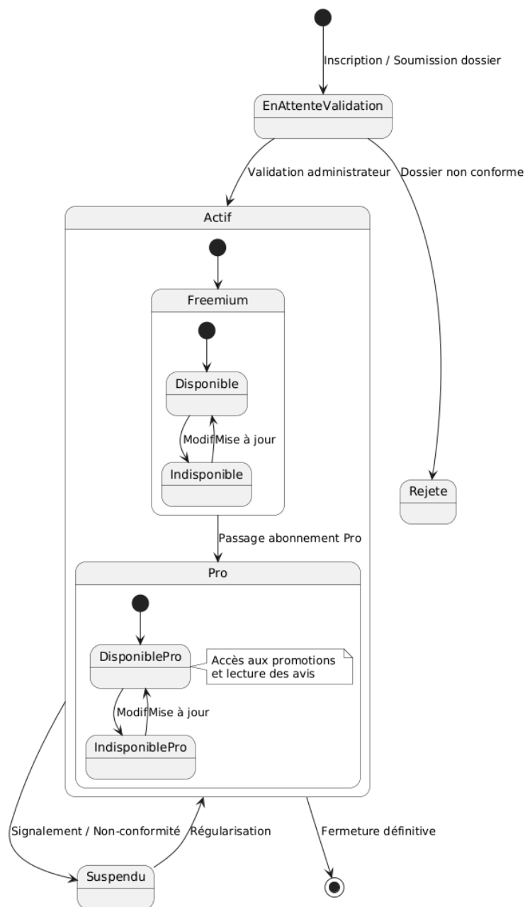
Figure 10: Diagramme d'état de cas gérer un établissement
